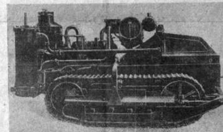
Tractor "oruga" Renault a gasógeno.
