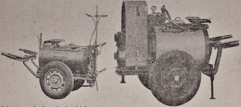
«Toboggau» es el pulverizador de calidad para viña.
