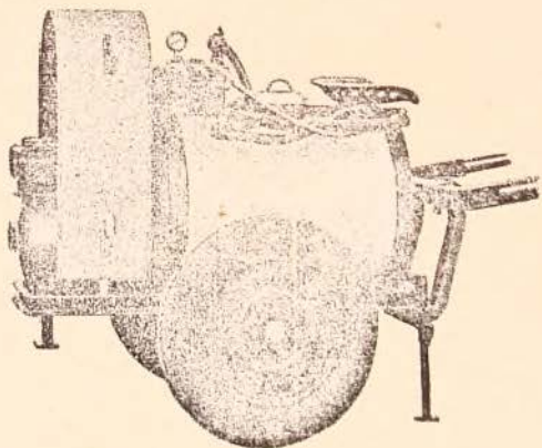
Pulverizador de alta precisión de los establecimientos Berthoud (Francia). La máquina para monte y viña. 200, 400 y 600 lit.
