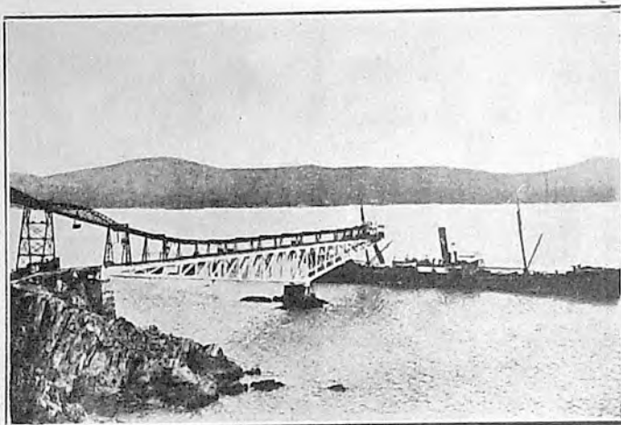
VIVERO. — Cargadero de la Mina de Hierro
