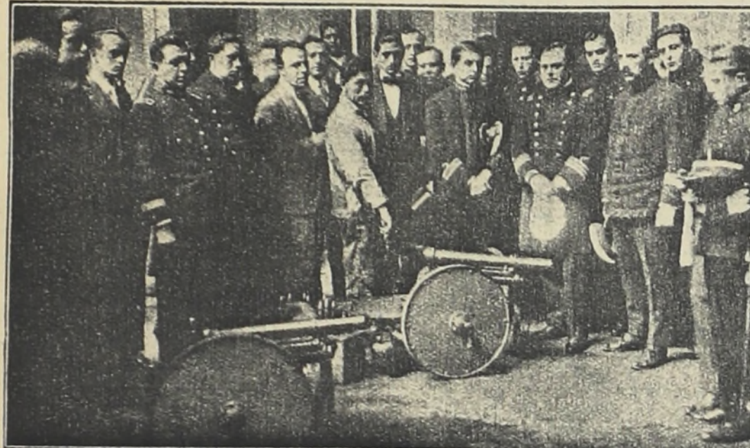
Cañón de campaña sistema Malpica inventado por un distinguido oficial mexicano y fabricado en ese país
