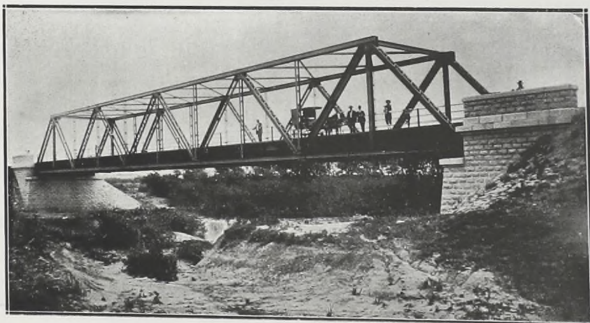
Puente sobre el Arroyo Agua Sucia
