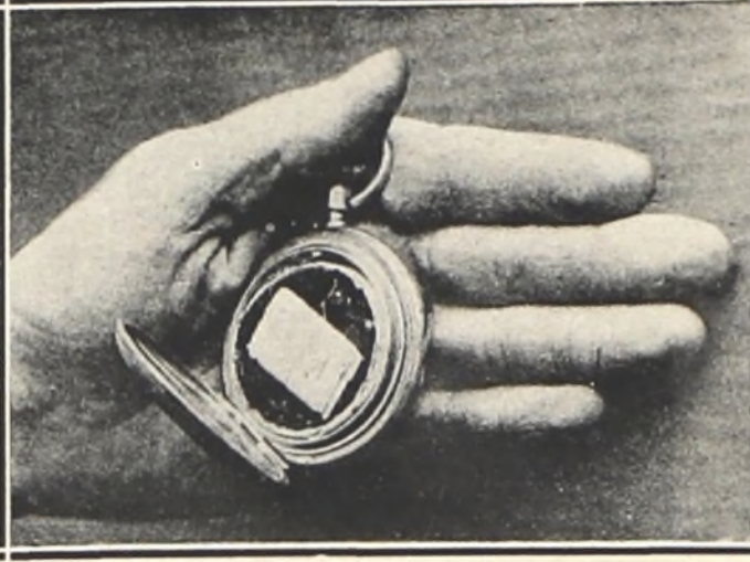
Pequeño receptor radiotelefónico, metido dentro de la caja de un reloj de tamaño normal, que puede usarse perfectamente
