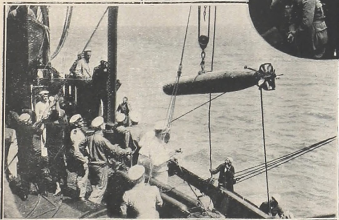
El torpedo de regreso del tiro, listo para ser embarcado
