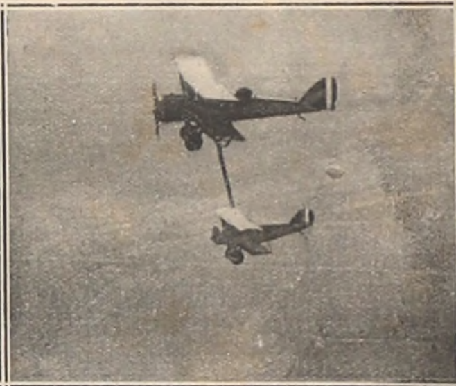
Un aeroplano del ejército norteamericano provee a otro de bencina a muchos metros de altura y sin detener el vuelo
