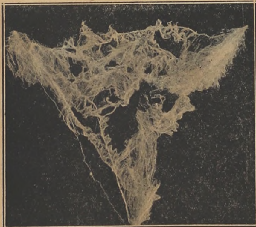
Una "corriente de ruptura" de un millón y medio de volts, fotografiada en el laboratorio de la General Electric Co. en sus talleres de Pittsfield
