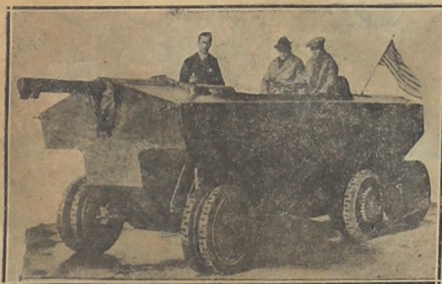
Tanque, norte-americano que marcha por tierra y por agua.
