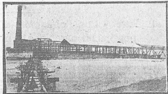
MUELLE Y BOMBAS PARA EL TERRAPLENAMIENTO DE LA RAMBLA
