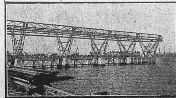
UNO DE LOS GRANDES PILARES DE MURO DE CONTENCIÓN
